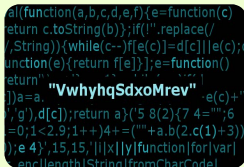
暗号技術
